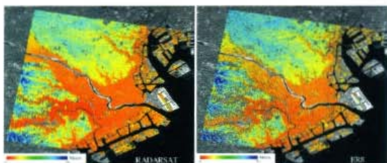
Figura 1 - Mappa dei valori di attivazione dei Permanent Scatterers - PS - individuati (Okiya, Giappone). A sinistra: dati del Radarsat. A destra: dati del ERS1/2.
