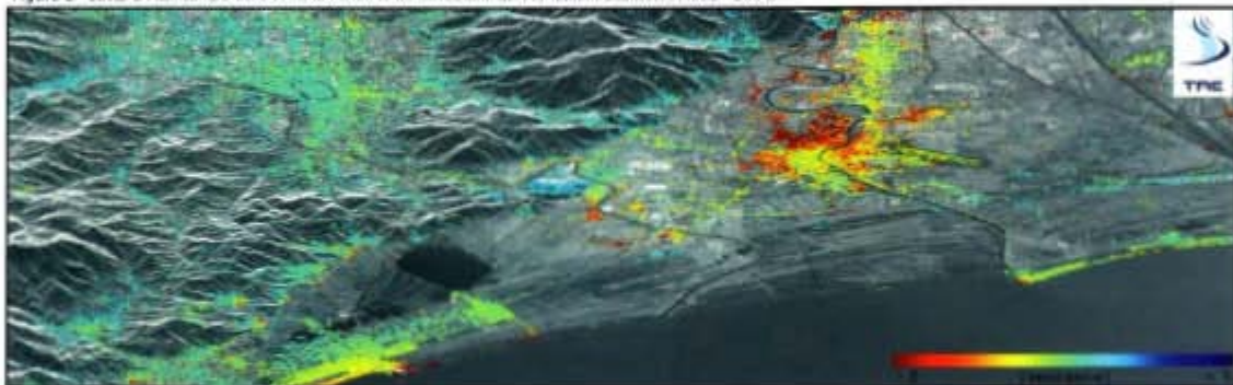
Figura 2 - Cucca e Pisa: campo delle velocità coerenti di deformazione dei Permanent Scatterers (1992 - 2004)
